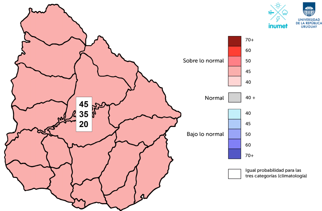
FIGURA 3 Probabilidades en porcentajes de los terciles de temperatura. Meses: marzo – abril – mayo de 2026.
