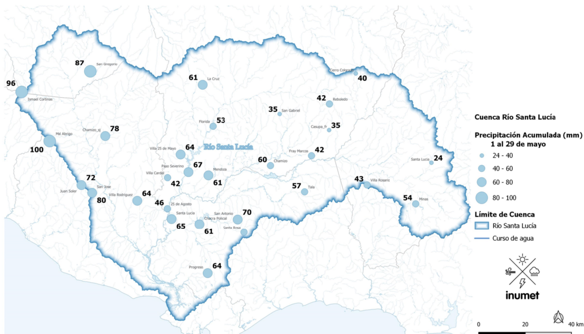
Figura 4 - Acumulados de precipitación del 1 al 31 de mayo en la cuenca del Santa Lucía.
