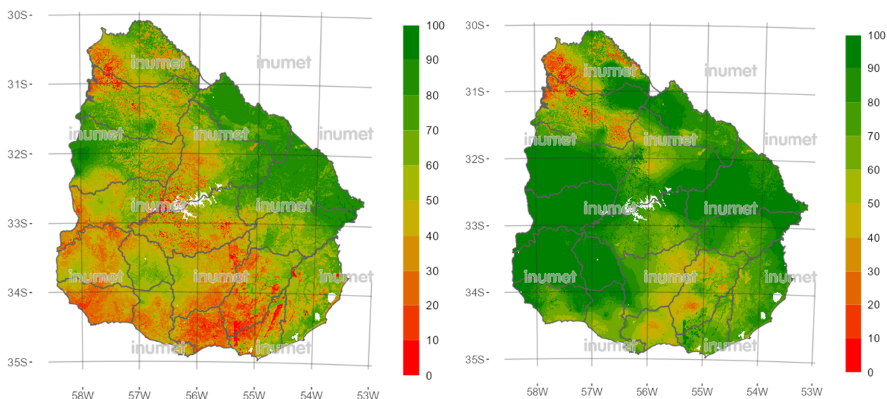
Figura 3 - Porcentaje de agua disponible en el suelo (%) al 20 de mayo (izq) y al 31 de mayo de 2023 (der).
